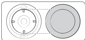
Tête du brûleur
